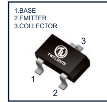
SOT-523
