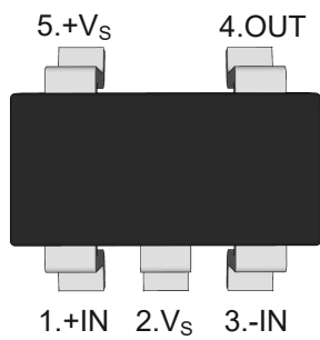
SOT-23-5
