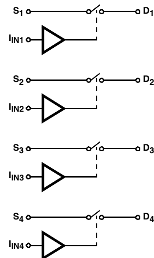
TRUTH TABLE
