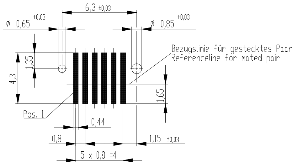
Leiterplatten-Layout Vorschlag PCB-Layout Proposal
