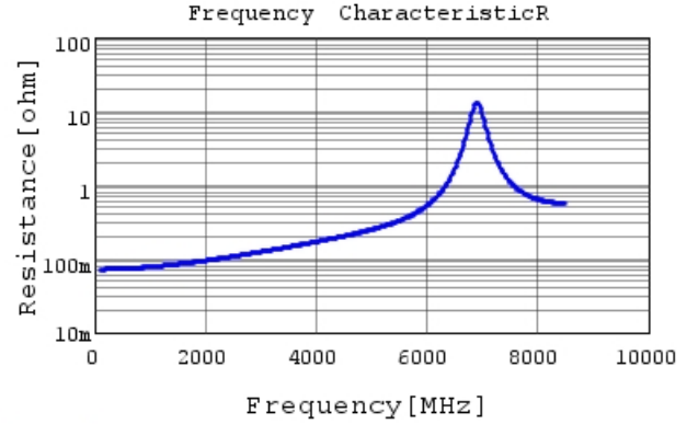
GCQ1555C1H9R5DB01 R DC0V, 25degC
