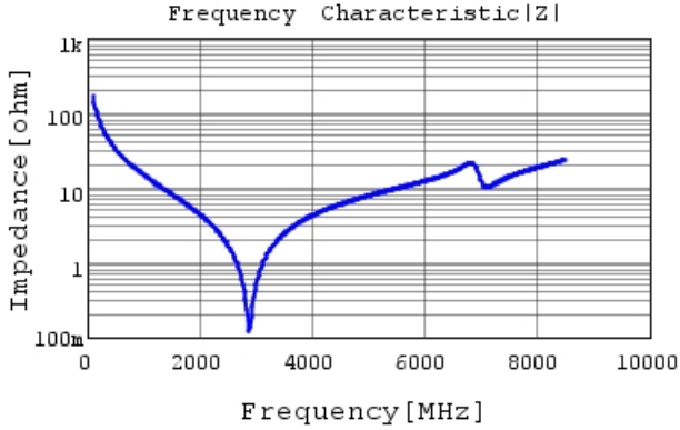
GCQ1555C1H9R5DB01 |Z| DC0V, 25degC
