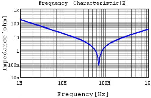
RCE7U2E102J1M1H03A |Z| DCOV, 25degC
