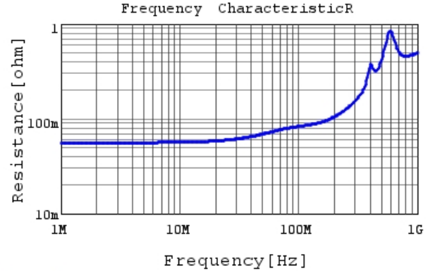
RCE7U2E102J1M1H03A R DCOV, 25degC
