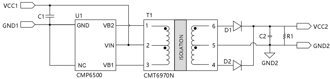
图 8.2 设计原理图
