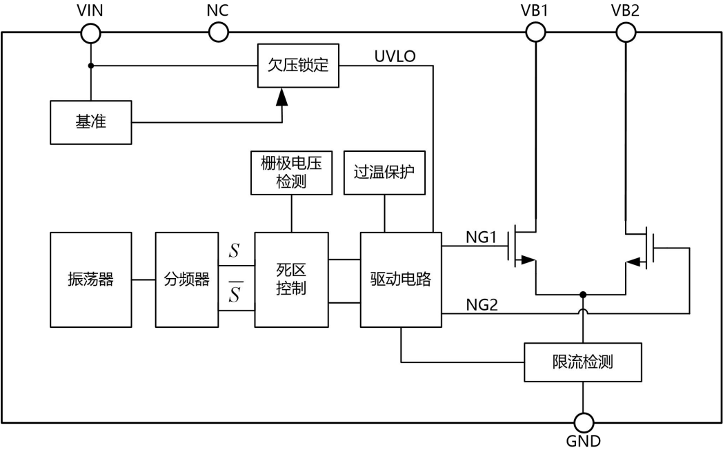
图 8.1 原理示意图
