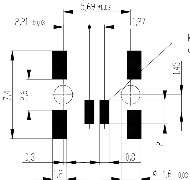
Leiterplatten-Layout für SMT PCB-Layout for SMT
