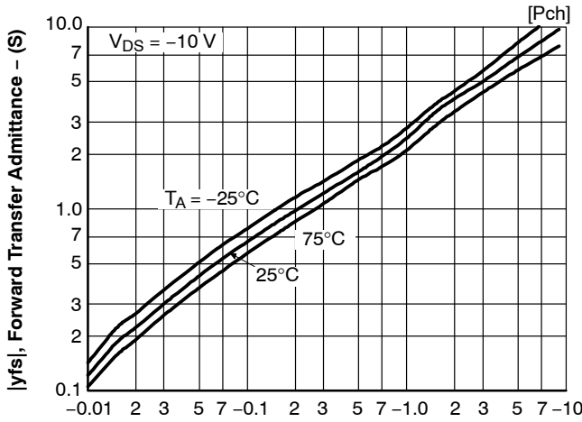
Figure 16. |y_{fs}| - I_D
