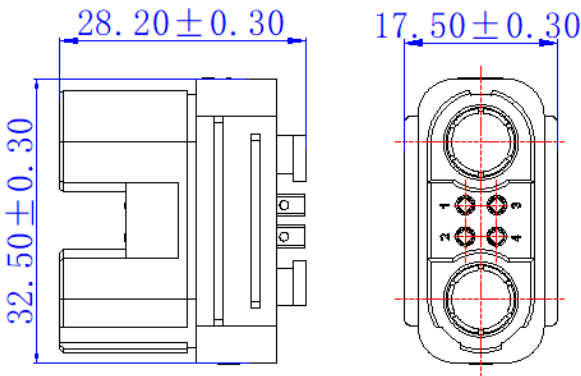
互配尺寸
