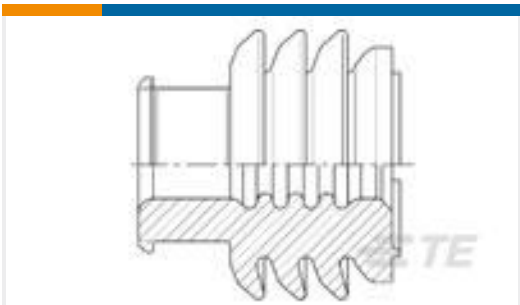
TE Part #1355437-2 MCP9,5 EINZELDICHTG
