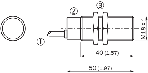
尺寸图 (尺寸单位: mm)
