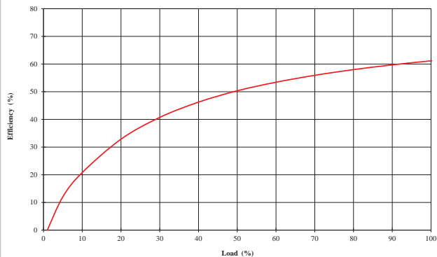
5V Input
