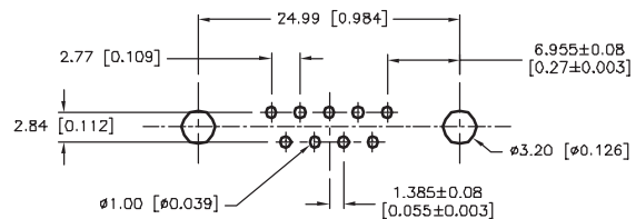
P.C.B. LAYOUT
