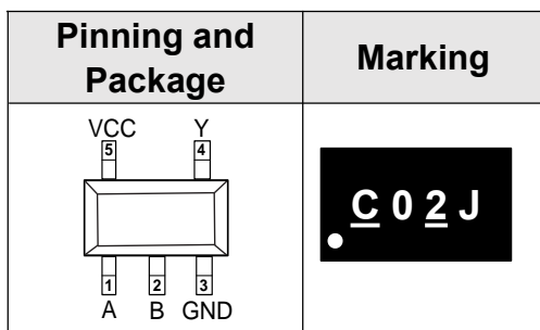
SOT23-5
