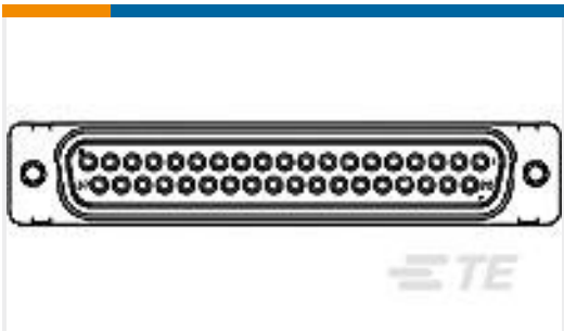
TE Part #1484950-1 AMPLIMITE PLG ASY,25P,SZ3,SER109
