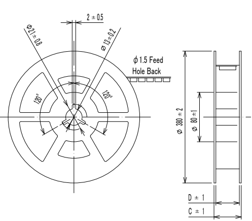
Reel Dimensions
