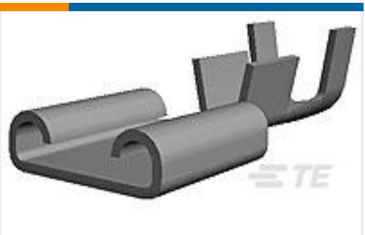
TE Part #2-160304-4 250 FASTON,REC.,14-17AWG,PNIPST
