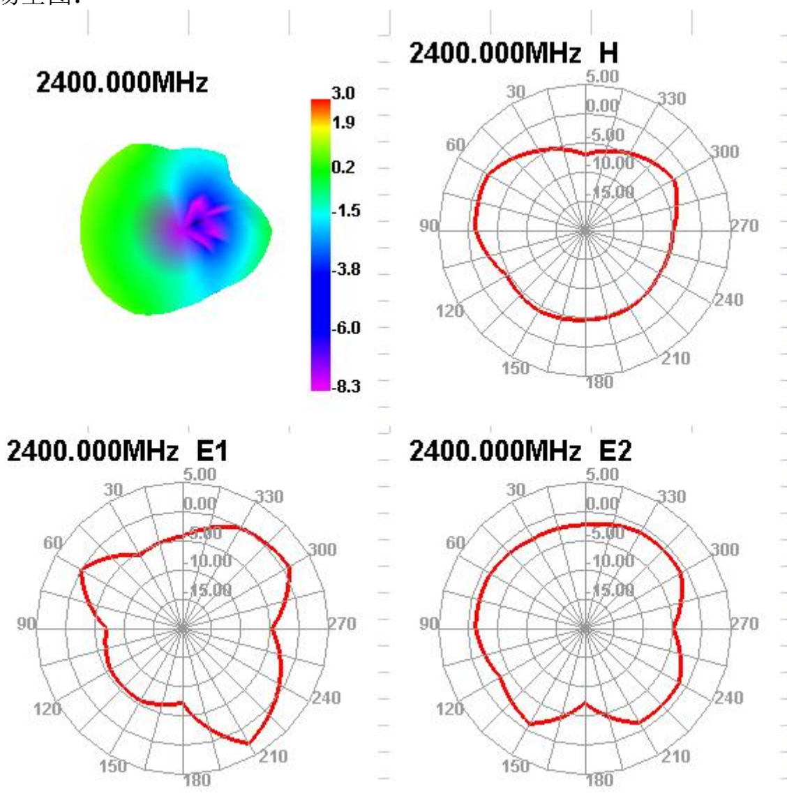
场型图:
