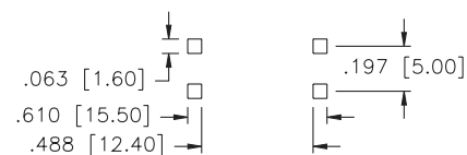
P.C. LAYOUT
