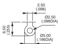
Solder lug
