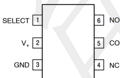
SOT363
