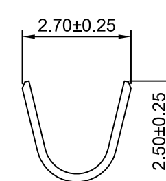
SEC:A-A
