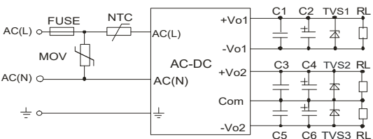
图3:CFAE20-T系列(三路)典型应用电路
