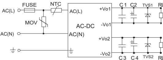
图4:CFAE20-DI系列(双隔离双路)典型应用电路
