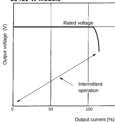
30-/50-W Models
