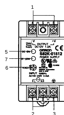
S82K-015□□
