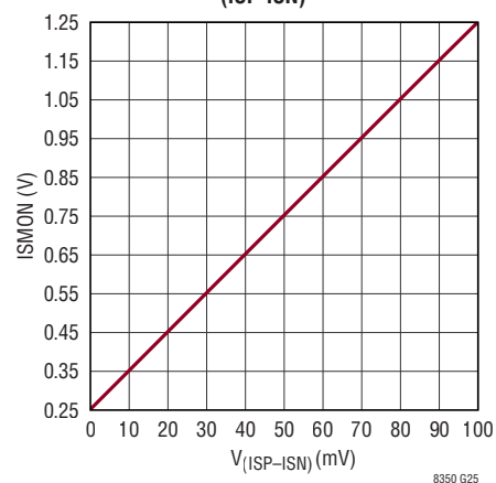
ISMON vs V_{(ISP-ISN)}
