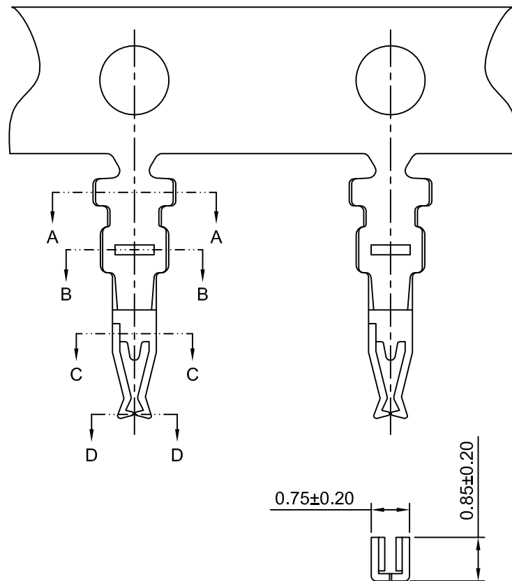
SEC:D-D
