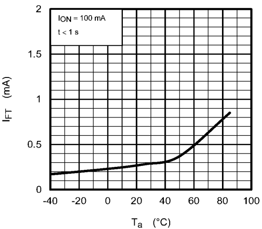
Fig. 13.1.6 I_{FT} - T_a
