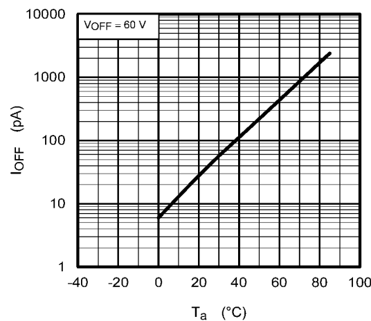
Fig. 13.1.10 I_{OFF} - T_a
