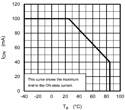
Fig. 13.1.2 I_{ON} - T_a
