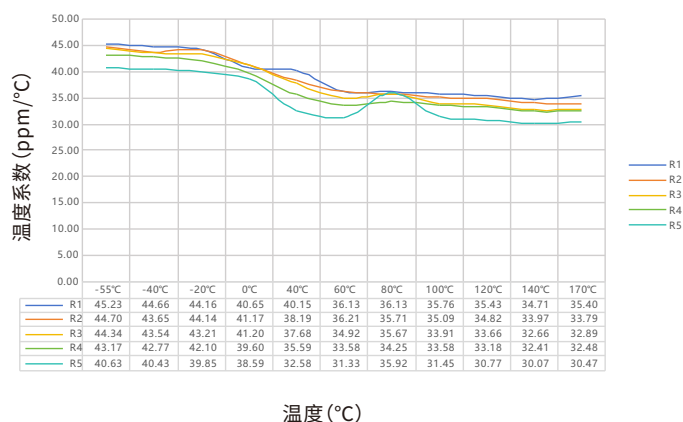
PEWK3920系列1.0mΩ温度系数实测数据表
