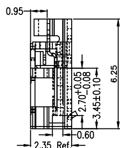
SEC A-A
