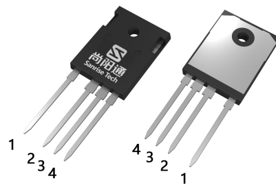
TO-247-4
