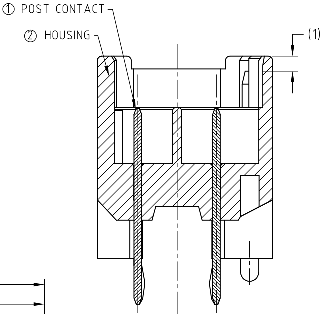
SECT A-A
