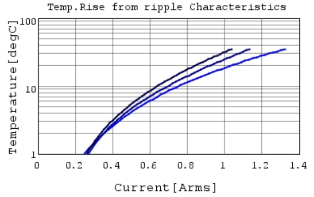
GRT1555C1E680JA02 Temp.rise — 200MHz
