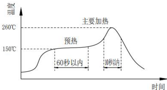
图 8. 回流炉温度设置条件
