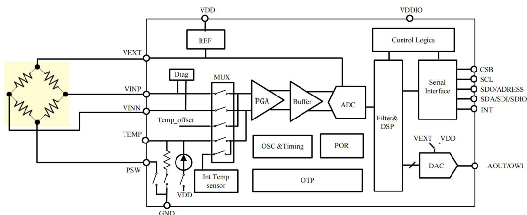
图 2 传感器功能框图
