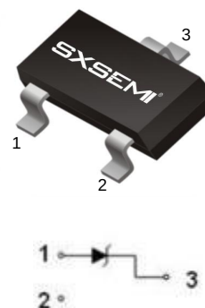
SOT-23
