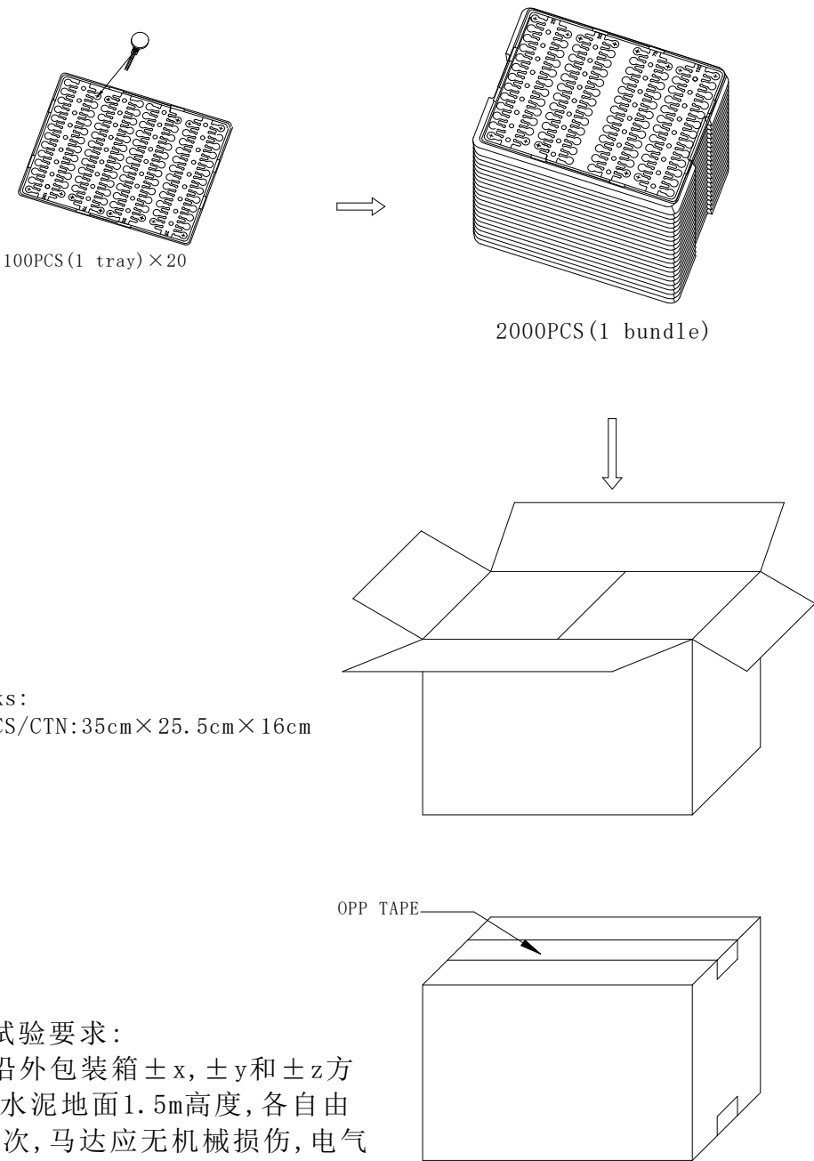
扁平系列马达包装 Pack drawing of coin type
