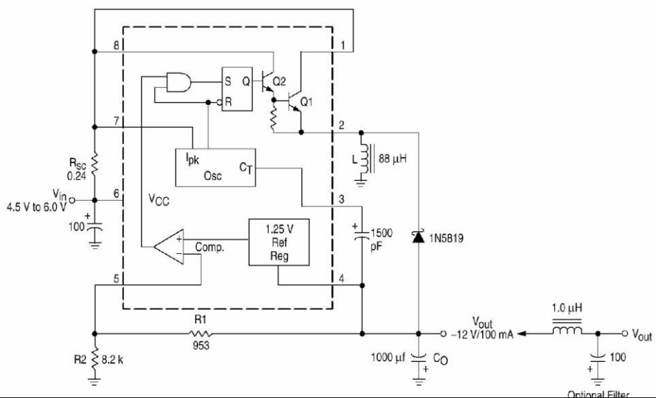
MC34063ADR2G 作反转式DC-DC 变换器
