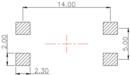
PCB.焊接图
