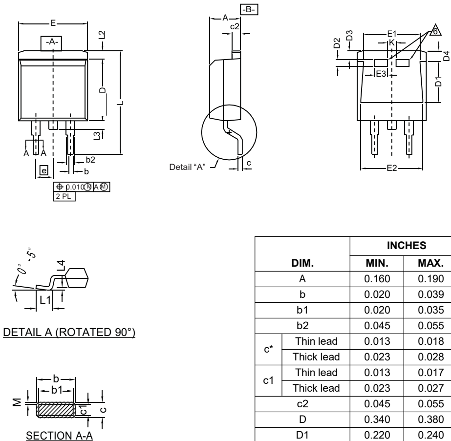
SECTION A-A
