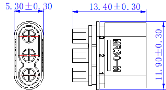
带后盖堆叠尺寸
