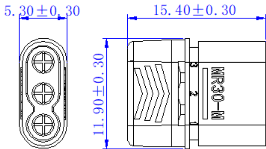
互配尺寸
