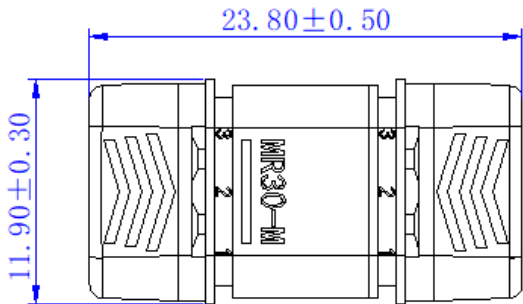
带后盖互配尺寸
