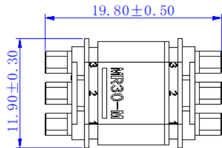
带后盖互配尺寸
