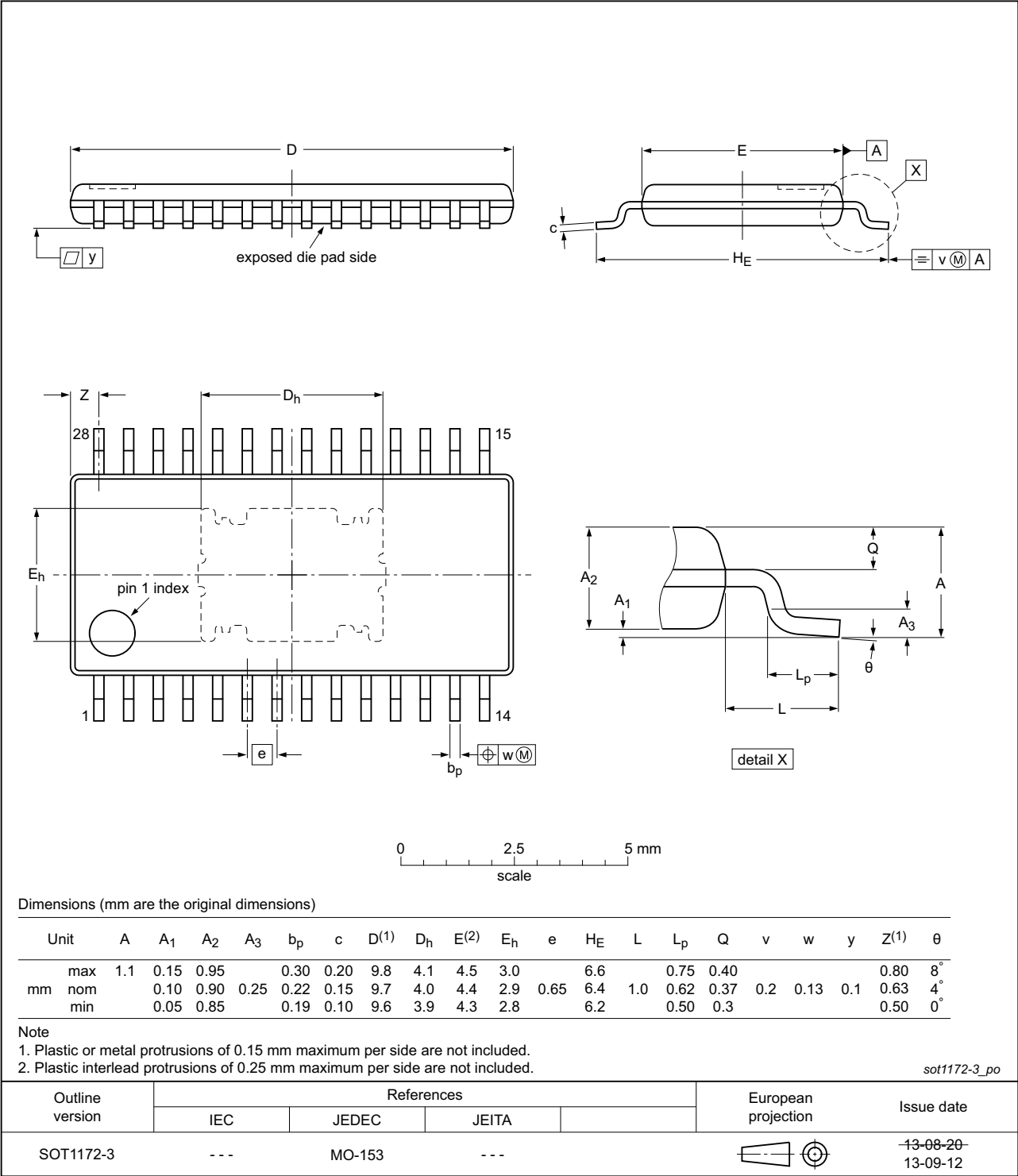
Fig 29. Package outline SOT1172-3 (HTSSOP28)
