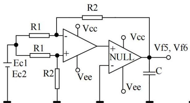
输入偏置电流 IBA 测试图
