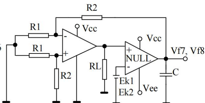
输入偏置电流 IBA 测试图
