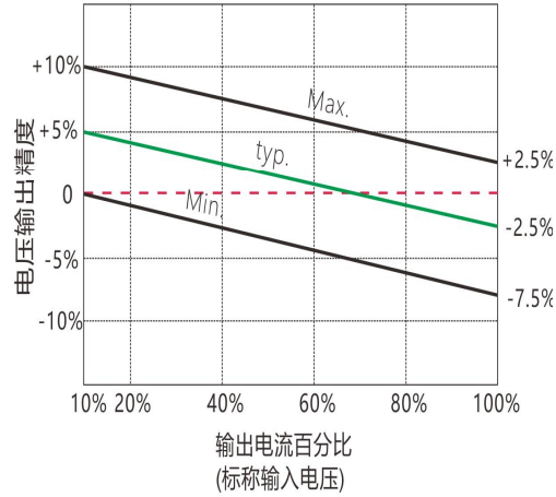
3.3VDC/5VDC输入/其他输出 误差包络曲线图
