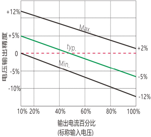
5VDC/12VDC/24VDC输入/3.3VDC输出 误差包络曲线图
