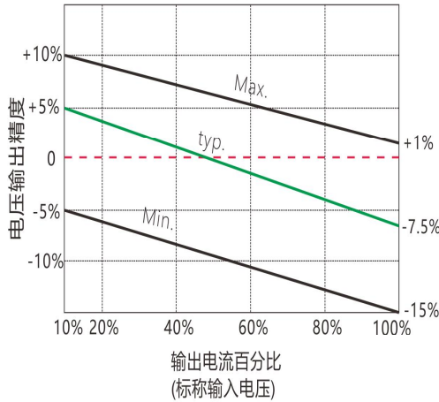
3.3VDC输入/3.3VDC输出 误差包络曲线图
