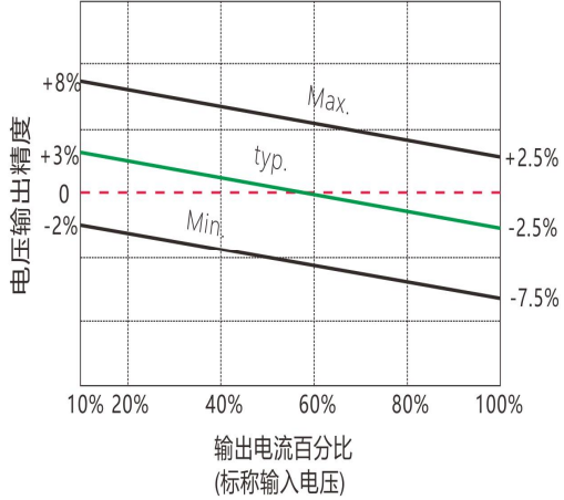
12VDC/15VDC/24VDC输入/其他输出 误差包络曲线图
