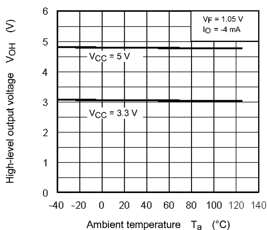
Fig. 12.2.4 V_{OH} - T_a
