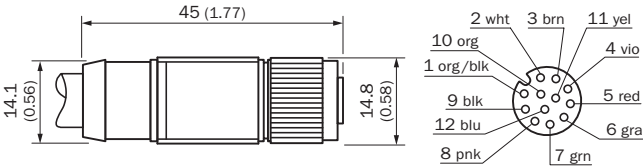
尺寸图 (尺寸单位: mm)
