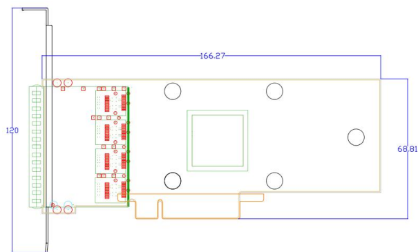
产品结构图
