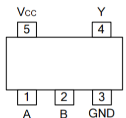
SOT23-5/ SOT353
