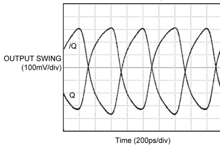
1.25GHz Output
