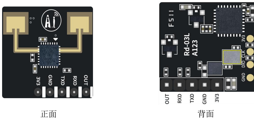
图 6 管脚示意图
