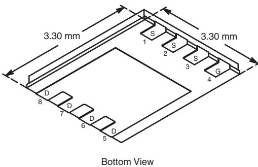
PowerPAK 1212-8
